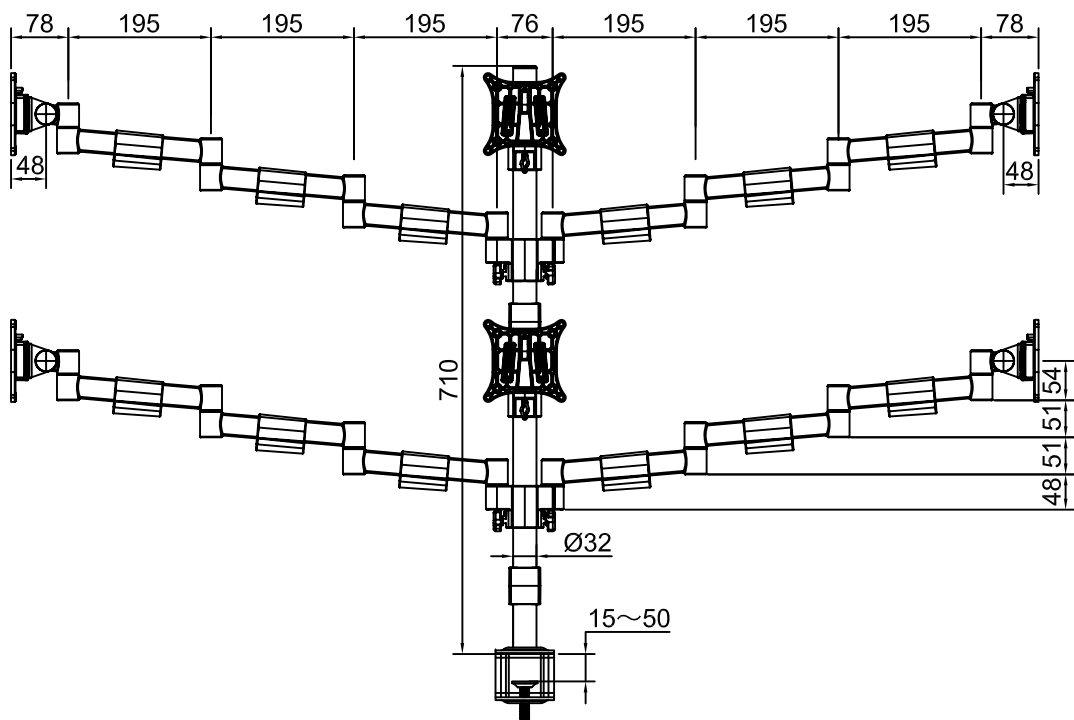
产品参数图
