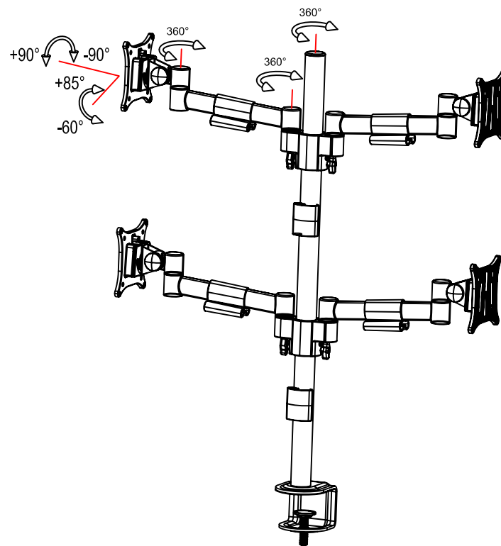
多功能调节示意图
